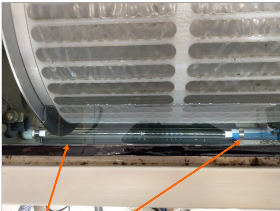
Den rostfria plåten och UV- rörets clips som popnitats fast
