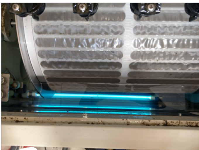
UV- röret ett par centimeter från trumman.
