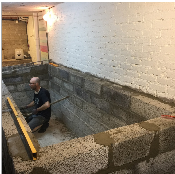
Rensning av fogarna för ett slätt underlag under gummiduken. (Man kan inte ha för många vattenpass när man gör en damm...)
