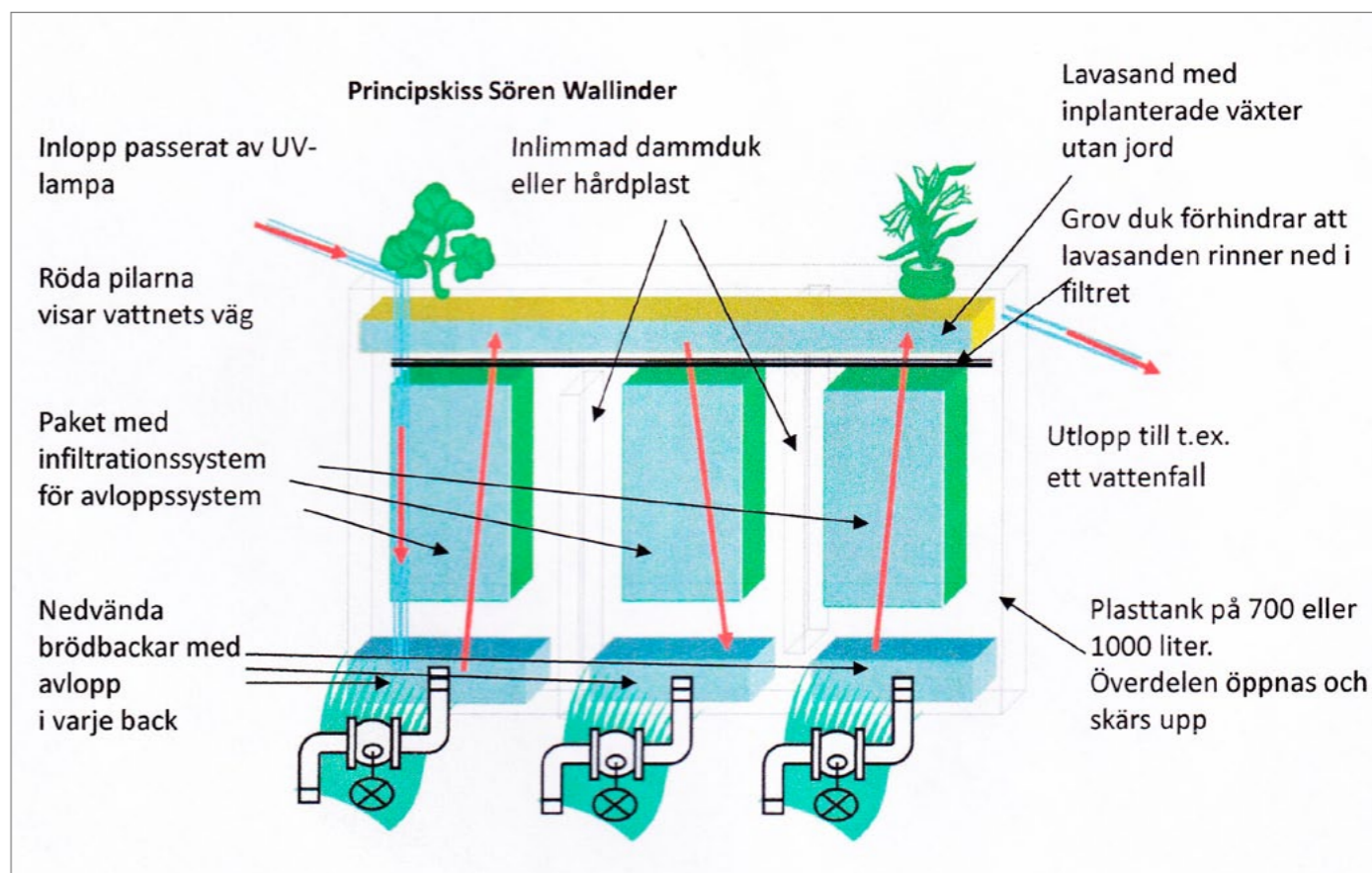
Skiss på Sörens reningsanläggning för den som kanske känner för ett nytt projekt framöver.
