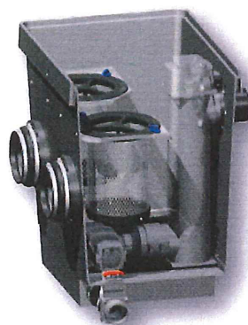
Individuell modul
